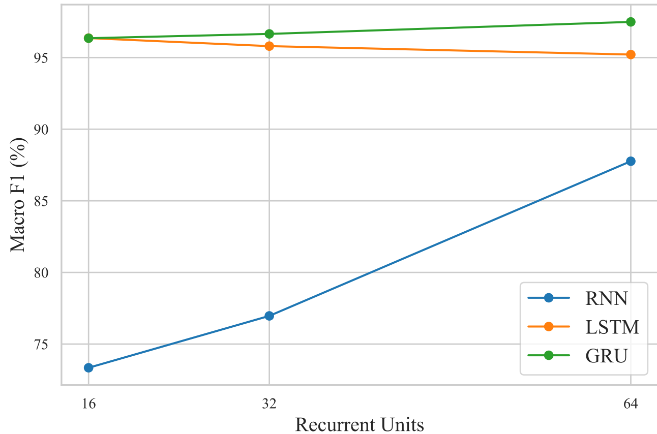
Recurrent Units vs. Test Macro F1
